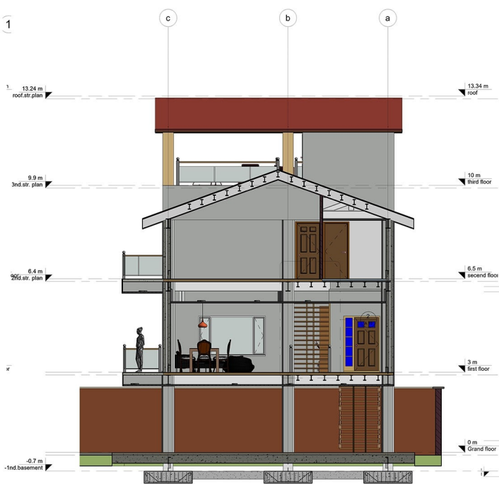
2 Section 2 1 : 50
